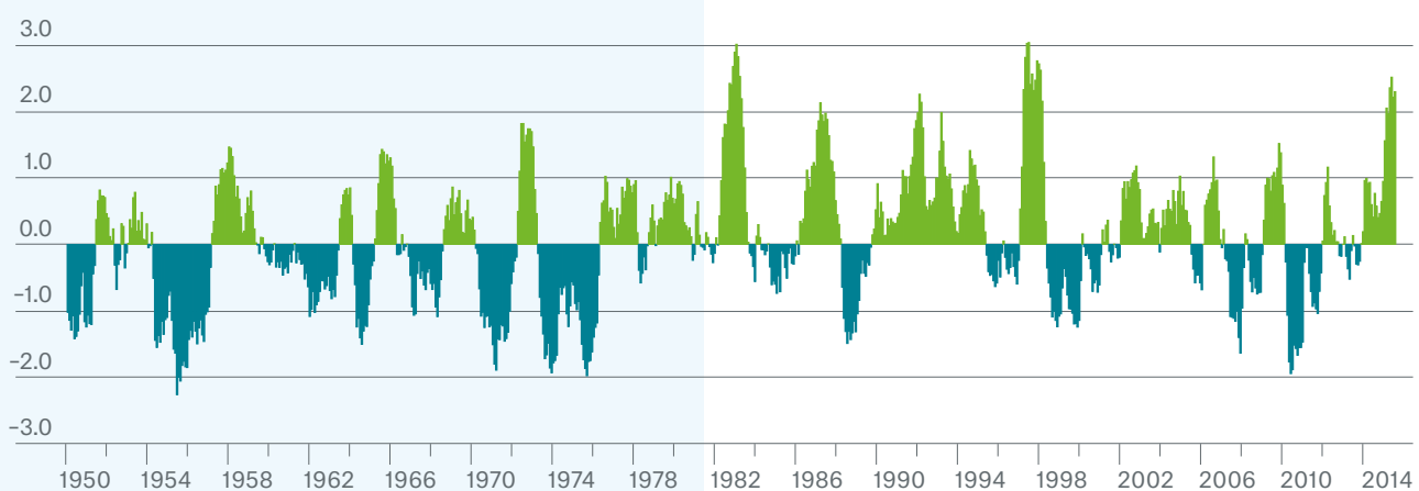
Multivariate ENSO Index
